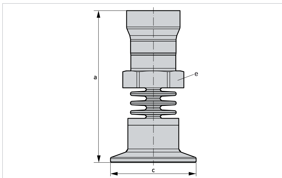
Figure 2-6: Clamp DIN 32676 / ISO 2852
